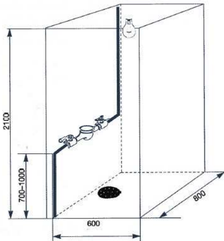
Fig. 5. För att komma åt vattenmätaren för avläsning eller service måste det finnas ett fritt utrymme runt mätaren enligt denna figur. Alla mått i mm.
